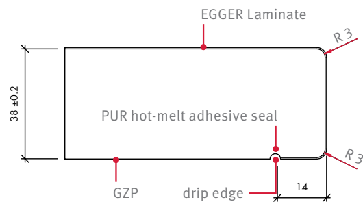
MODEL 300/3 DRIP EDGE
